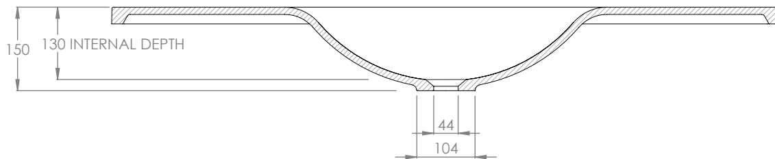
SECTION A-A
